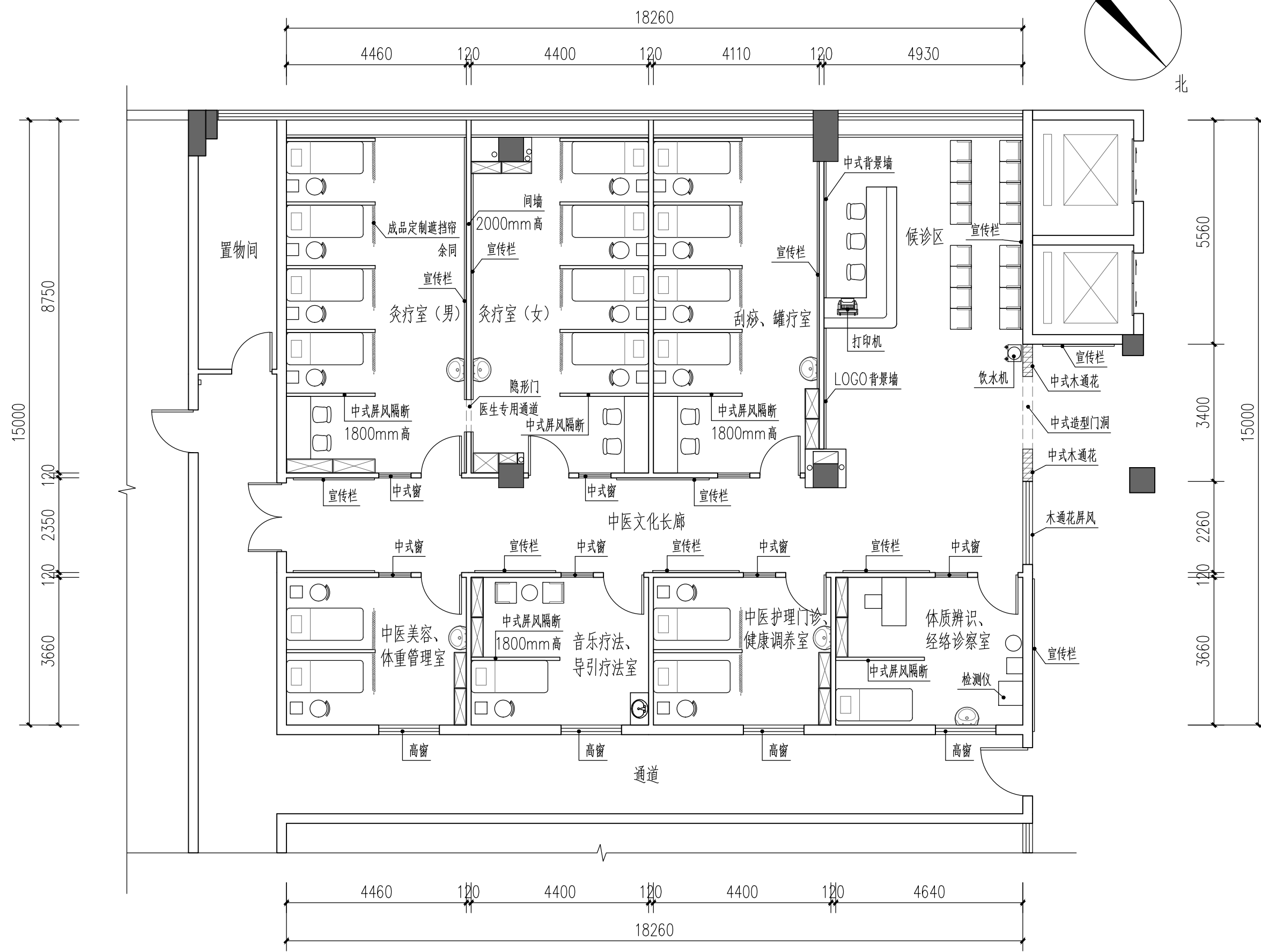
平面布置图 1:100
