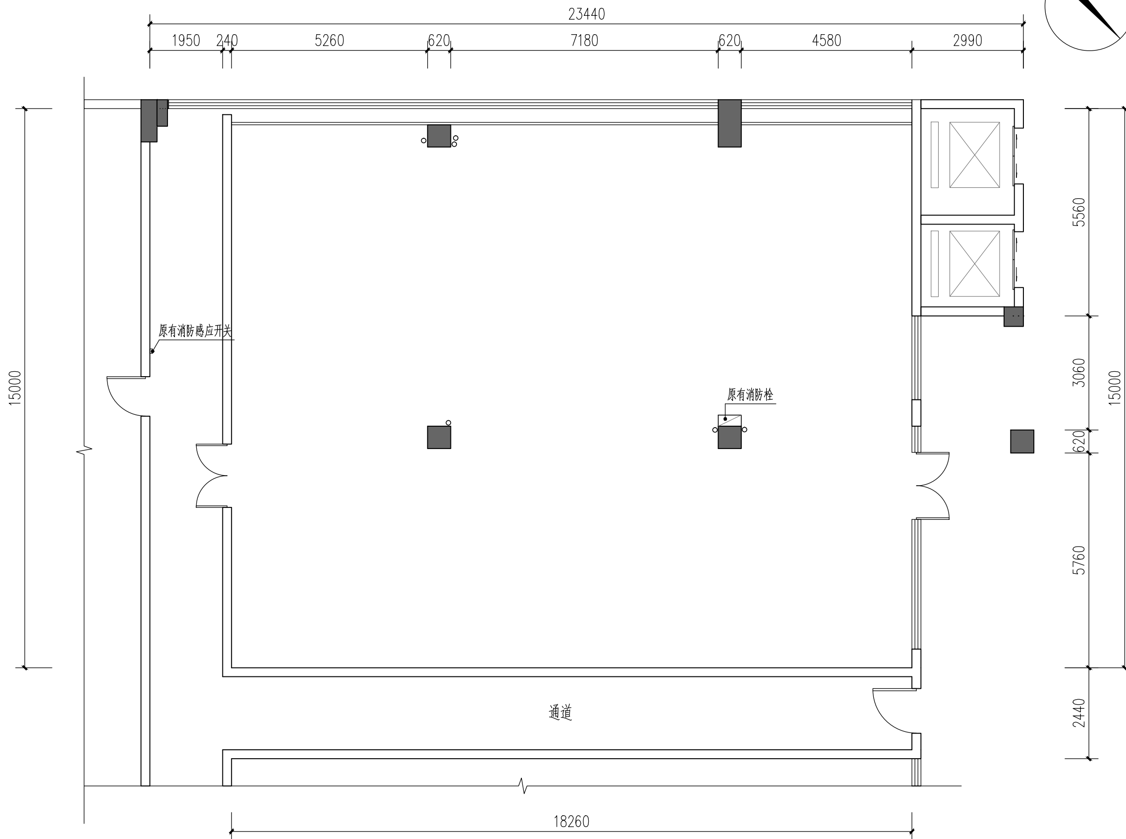
原始平面图 1:100
